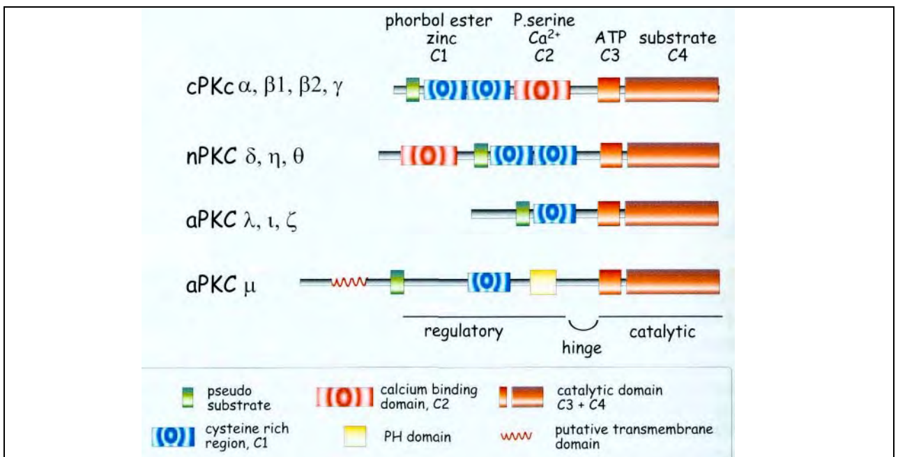
Рис.7.2 Доменная структура семейства протеинкиназ С. Семейство протеинкиназ С млекопитающих состоит из 12 членов разделенных на 3 подсемейства: обычные (с), новые (н) и атипичные (а). Они отличаются консервативными доменами C1, C2, C3, и C4. Белок состоит из регуляторных и католитических доменов, соединенных шарнирными областями (1 группа протеинкиназ: альфа, бета, гамма; 2- дельта, эта, тэта;
