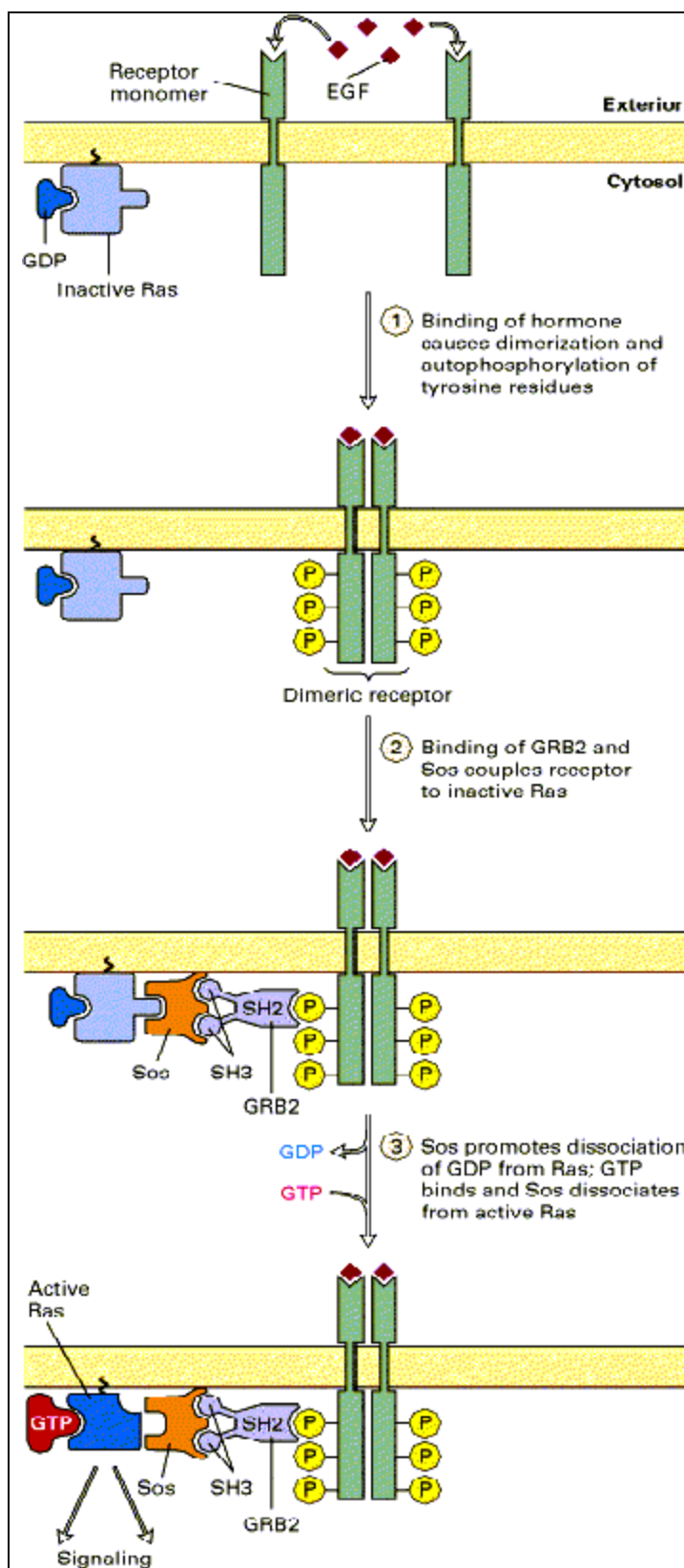
Рис.2.7 Активация Ras при связывании EGF с тирозинкинасным рецептором (ТКР).
