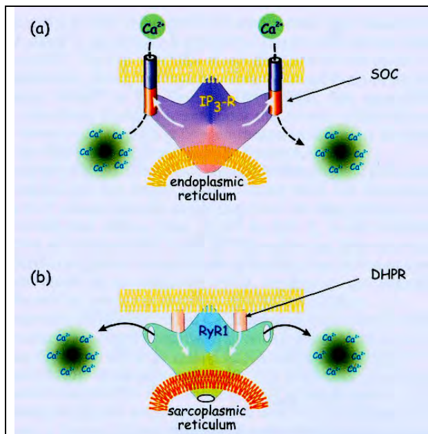
Рис.6.5 Сопряжение рианодинового и IP 3 рецепторов с каналами плазматической мембраны. Модель предполагает, что конформационные изменения в IP 3 R (a) и RyR (b) могут индуцироваться прямым взаимодействием с белками – каналами плазматической мембраны. (a) – Депо-зависимые каналы (SOC) и (b) - дигидропиридиновый рецептор (DHPR)
