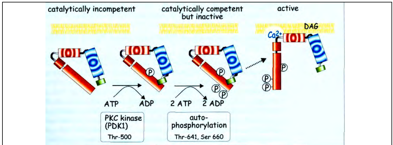
Рис. 7.3 Активация протеинкиназы С (PKC) требует фосфорилирования каталитического домена и отсоединения псевдосубстрата. Активация PKC происходит в 4 ступени. PKC синтезируется как предшественник 74 кДа. Исходно ее каталитический участок доступен для субстрата, но не активен. Далее следуют три различных фосфорилирования, переводя фермент в каталитически компетентное, но еще не активное состояние. Возможно, это делает PDK1-фосфолипид-зависимая киназа. Доступ субстрата предотвращается присоединением псевдосубстрата (зеленый) к каталитическому участку (красный). При связывании DAG и увеличении Ca^{2+} фермент прочно связывается с мембраной, псевдосубстрат отсоединяется от каталитического участка и он становится доступным для субстрата готов к фосфорилированию.
