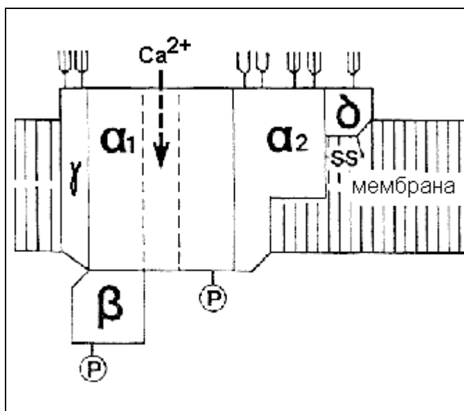
Рис. 6.1 Субъединичная структура потенциал-управляемого кальцевого канала. Указаны места фосфорилирования (P), гликозилирования (Ψ, Υ) и дисульфидный мостик (-SS-).
