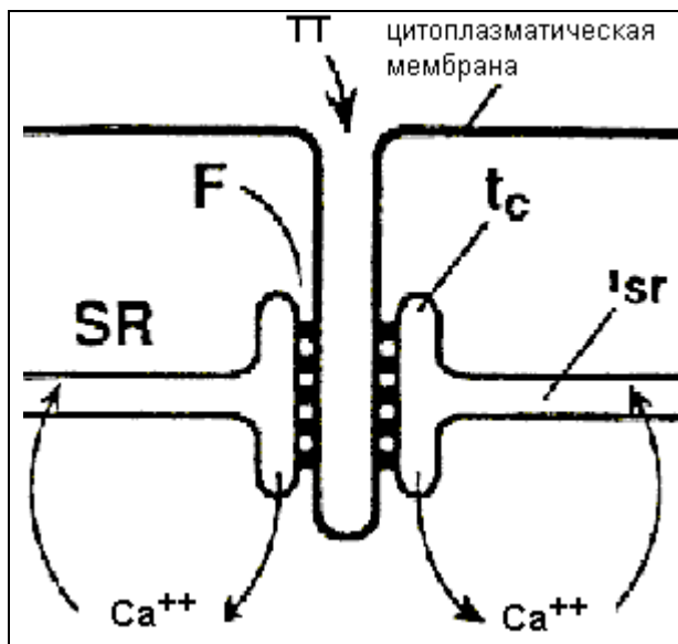
Рис. 6.3 Схема контакта между цитоплазматической мембраной (сарколеммой) и сарко/эндоплазматическим ретикулом. ТТ (transverse tubule)- поперечная трубочка, SR - саркоплазматический ретикулум, tc - терминальная цистерна, l sr - продольная трубочка SR, F - так называемая область "ножки" (foot-region).
