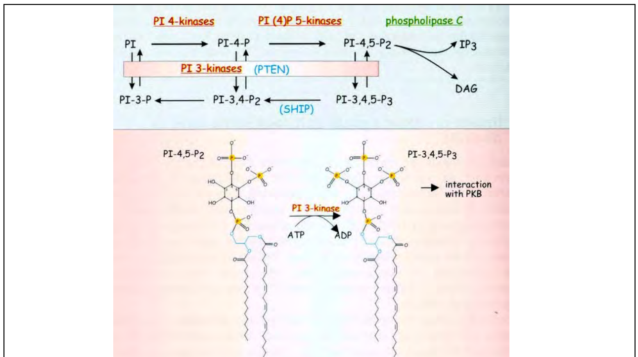
Рис. 7.8 Фосфоинозитид 3-киназы и генерация 3-фосфорилированных липидов.
