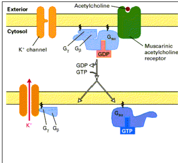
Рис. 2.10 Ацетилхолин (АХ) индуцирует открытие K + каналов в плазматической мембране клеток сердечной мышцы. Связывание АХ с мускариновым АХ-рецептором активирует обмен GTP на GDP на α субъединице G белка. Освобожденная βγ субъединица связывается с K + каналом и открывает его. Увеличение проницаемости для K + гиперполяризует мембрану, что уменьшает частоту сердечных сокращений.
