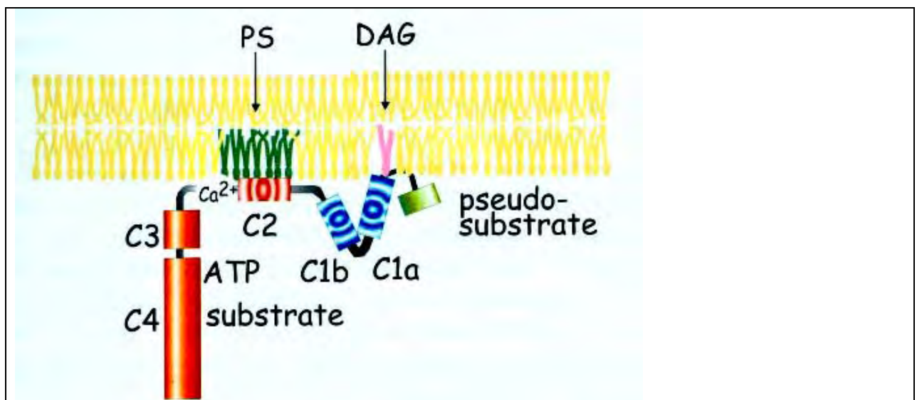
Рис. 7.4 Домены PKC. Консервативные домены C1-C4 являются функциональными модулями. C1 связывает DAG или форболовый эфир, C2 участвует в присоединении к отрицательно-заряженному фосфолипиду (фосфатидилсерин), которое усиливается связыванием Ca^{2+} . В некоторых изоформах присутствует это Ca^{2+} -связывающее место, ответственное за Ca^{2+} -зависимое связывание с липидом (PS). C3 и C4 являются каталитическими доменами. Шарнирное соединение между C1,C2 и C3,C4 при связывании PKC с мембраной становится легко доступной мишенью для протеолитических ферментов типа трипсина. Фрагмент, содержащий киназный домен открепляется от мембраны и постоянно активен.
