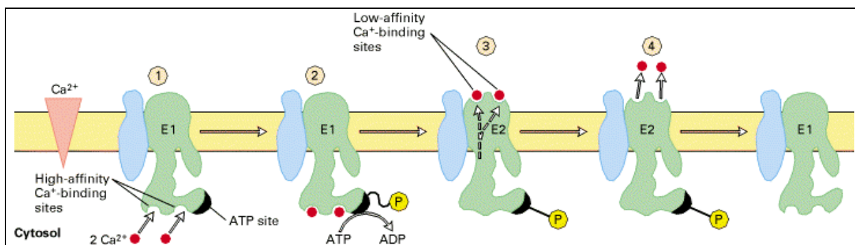
Рис.6.11 Модель механизма действия \text{Ca}^{2+} АТР-азы СР. Показана только одна из двух субъединиц. E1 и E2 являются альтернативными конформационными формами белка, в котором \text{Ca}^{2+} -связывающие участки находятся на цитозольной и внутренней поверхности ретикулярной мембраны соответственно. \text{Ca}^{2+} ионы (красные кружочки), \sim\text{P} обозначает высокоэнергетическую ацил-фосфатную связь, P – низкоэнергетическую фосфоэфирную связь. [адаптировано из работ W. P. Jencks, 1980, Adv. Enzymol. 51 :75; W. P. Jencks, 1989, J. Biol. Chem. 264 :18855; and P. Zhang et al., 1998, Nature 392 :835.]
