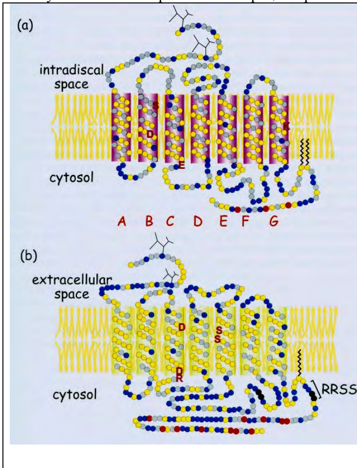
Рис 2.8. Расположение в мембране родопсинового и адренергического рецепторов. Мембранная организация (a) родопсинового и (b) \beta 2-адрено-рецептора. Обе структуры включают семь трансмембранных гидрофобных доменов (A-G). Остатки, вступающие в контакт с лигандами (I, цис-ретиналь и адреналин) обозначены отдельными буквами. Красным отмечены остатки – мишени фосфорилирования родопсинкиназой и \beta 2-адренорецепторной киназой. Остатки, отмеченные черным – мишени фосфорилирования РКА. Желтым цветом показаны гидрофобные остатки; серым - неполярные; красным - гидрофильные.
